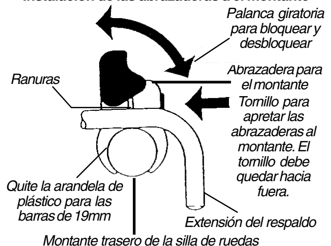
FIGURA 1 - INSTALACIÓN DEL RESPALDO ULTI-MATE EN LOS MONTANTES TRASEROS SUPERIOR INFERIOR
